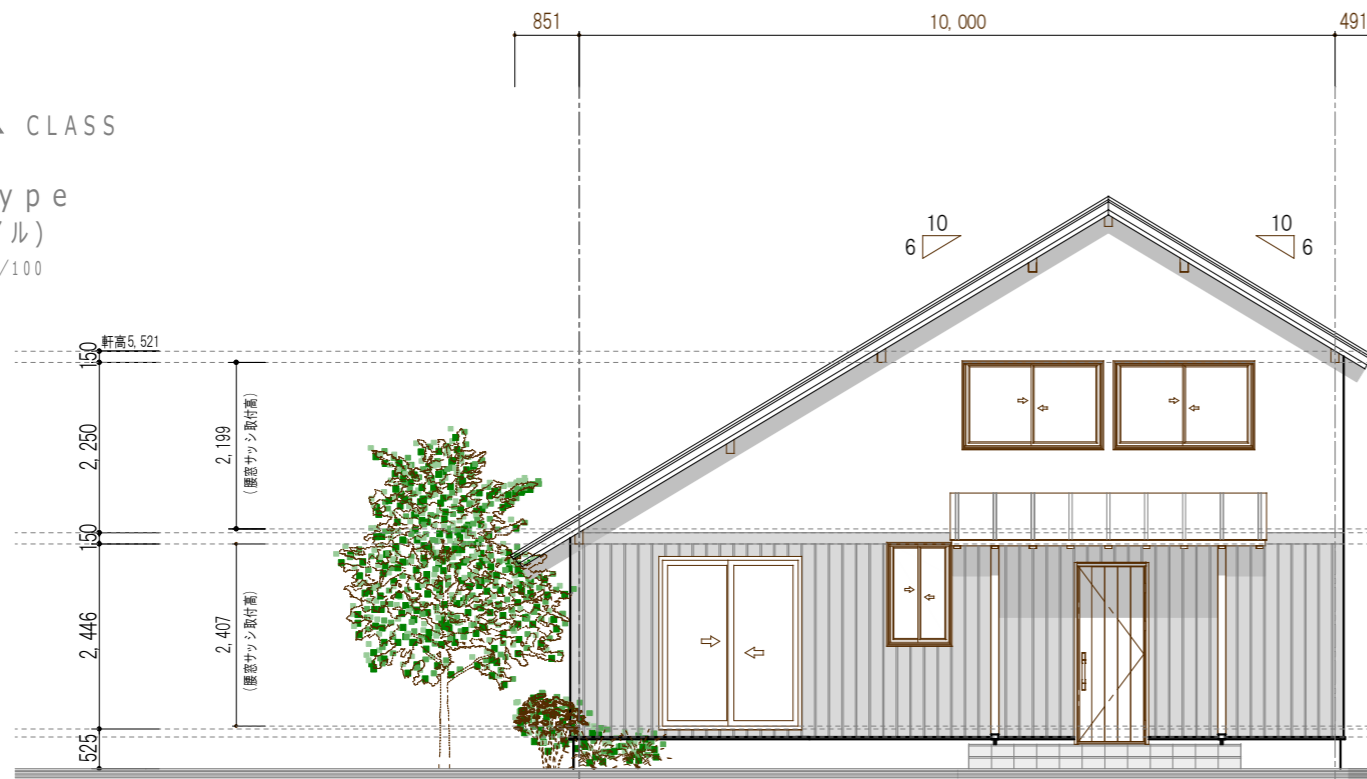
南立面図 S = 1 : 1 0 0
